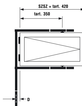
VENTUS F 200 ablaktávnnyító Nyílószárny T-sarokkal (lásd: Tartozékok oldal)
