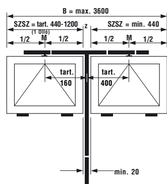
VENTUS F 200 ablaktávnnyító Duplaszárny nyitás 2n T-sarokkal (lásd: Tartozékok oldal)
