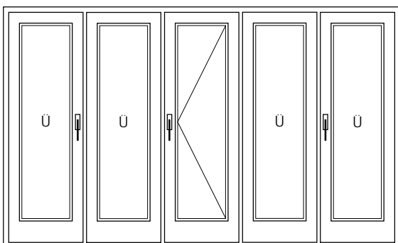
532 séma 4 harmonika szárny 1 nyíló szárny
