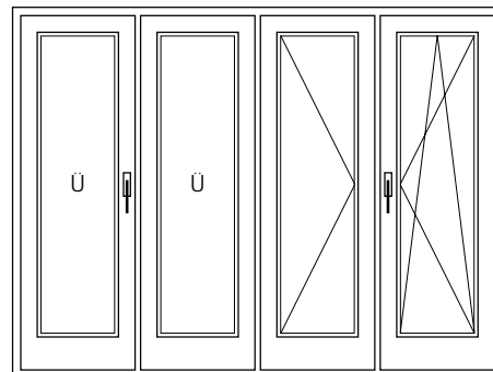
431 séma [1] 2 harmonika szárny 1 váltószárny, 1 bukó-nyíló szárny
