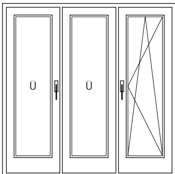
321 séma [1] 2 harmonika szárny 1 bukó-nyíló szárny
