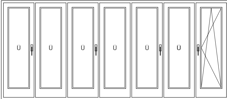
761 séma [1] 6 harmonika szárny 1 bukó-nyíló szárny
