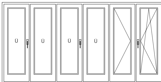
651 séma [1] 4 harmonika szárny 1 váltószárny, 1 bukó-nyíló szárny
