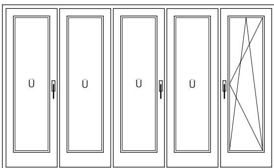
541 séma [1] 4 harmonika szárny 1 bukó-nyíló szárny
