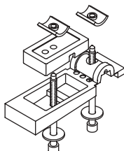
Alsó összekötő csomag SZV 56 mm K-11705-00-0-3 SZV 68 mm K-13113-00-0-3
