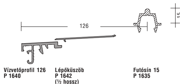
Lépőküszöb P 1642 (1/2 hossz)
