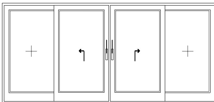
C séma 2 Emelő-toló ajtó, 2 Fix rész Ábra: Szárny perem balra és szárny perem jobbra
